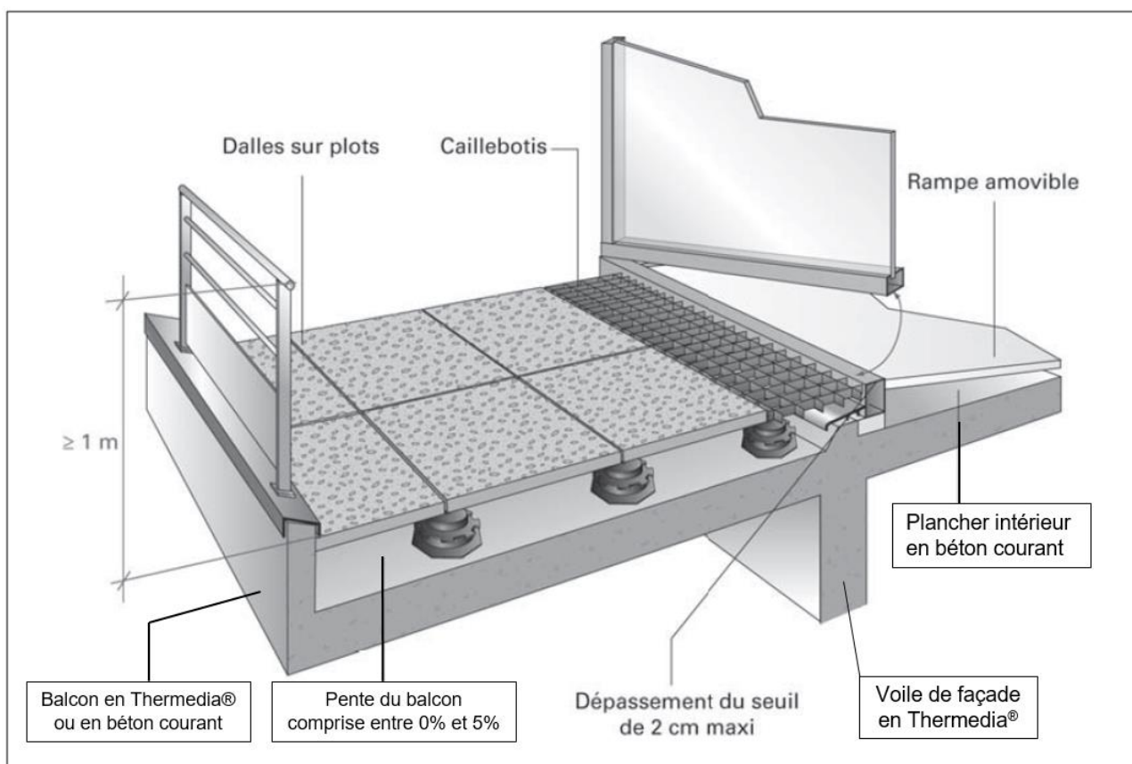
Figure n° E1 – Exemple de balcon, loggia ou coursive sans revêtement d'étanchéité – Garde d'eau assurée par un ressaut coulé en œuvre
