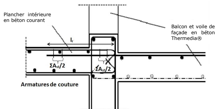
Figure 8 – Armatures de couture en cas de recouvrement à distance
