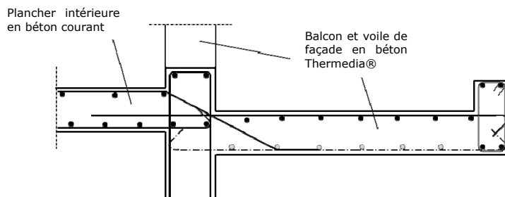
Figure 7 – Dénivellement a supérieur ou égal à 4 cm (dénivellement limité par une pente de 1/3 : voir § 2.3.4.2.6).
