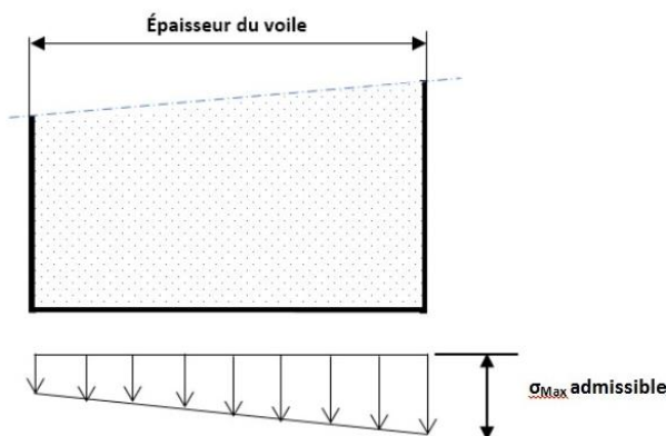
Figure 2 - Représentation de \sigma_{Max} admissible
