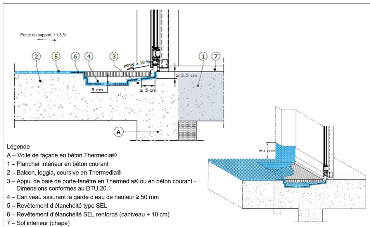
Figure n° E5-1 – Exemple de balcon, loggia ou coursive avec étanchéité par un S.E.L. directement circulaire - Seuil avec caniveau – 1,5 \% \leq pente \leq 5 \%
