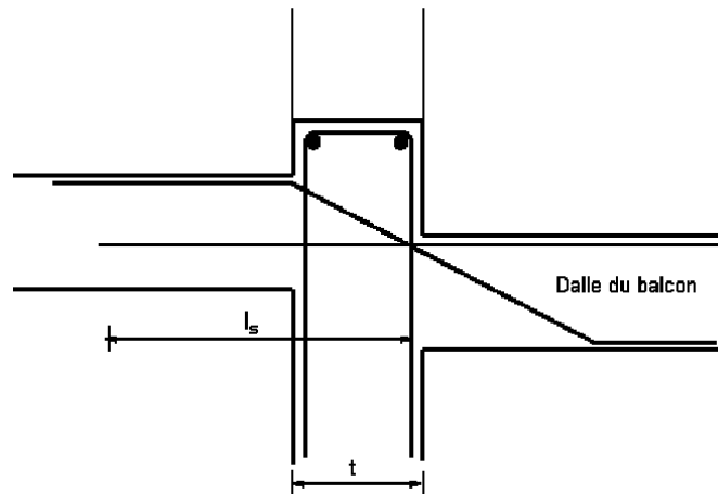
Figure 3 – Longueur d'ancrage L_s
