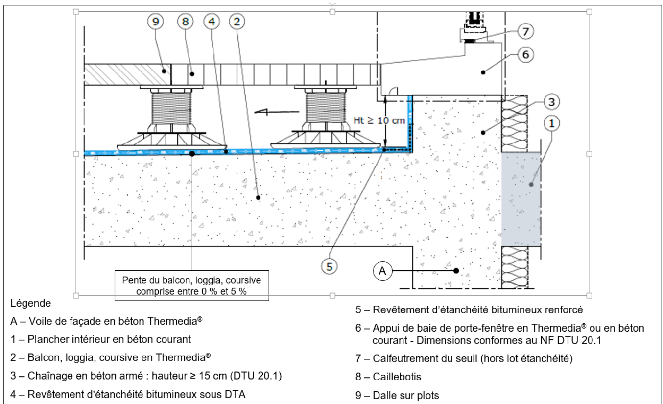
Figure n° E4-1 – Exemple de balcon, loggia ou coursive avec étanchéité par un revêtement bitumineux sous DTA avec protection par dalles sur plots - Seuil avec relevé de 10 cm de hauteur.
