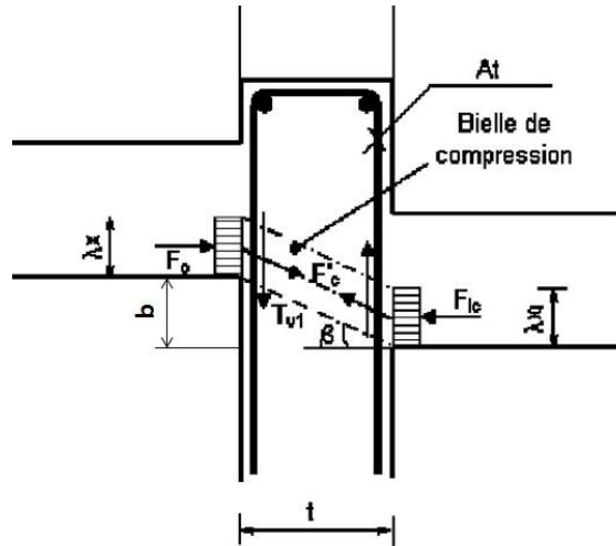
Figure 4 – Inclinaison des bielles de compression
