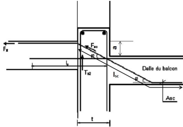
Figure 5 – Inclinaison des armatures à l'appui de la dalle du plancher intérieur
