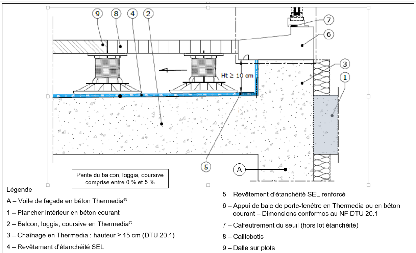
Figure n° E3-1 – Exemple de balcon, loggia ou coursive avec étanchéité par un S.E.L. avec protection par dalles sur plots - Seuil avec relevé de 10 cm de hauteur.
