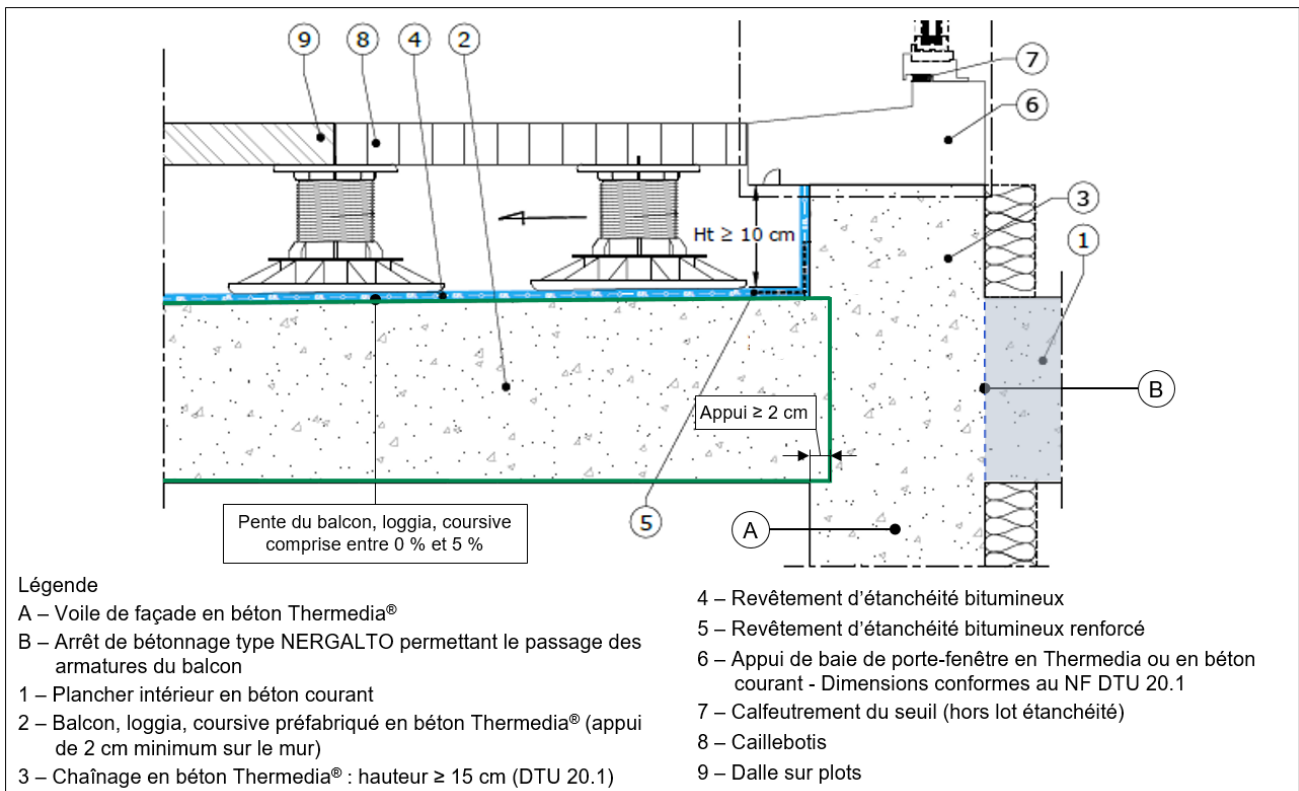
Figure n° E4-2 - Exemple de balcon, loggia ou coursive préfabriqué avec étanchéité par un revêtement bitumineux avec protection par dalles sur plots - Seuil avec relevé de 10 cm de hauteur.
