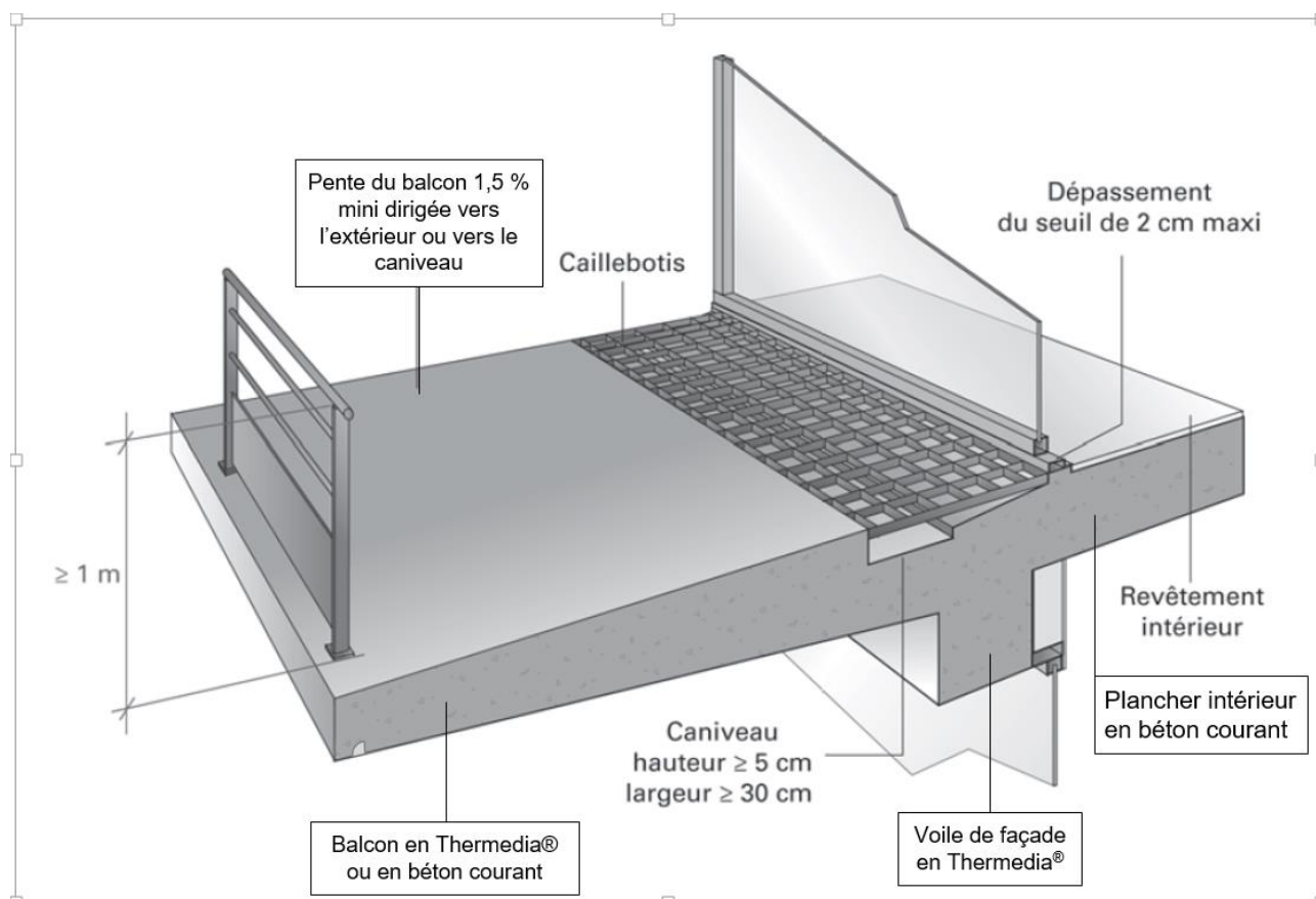
Figure n° E2 – Exemple de balcon, loggia ou coursive sans revêtement d'étanchéité – Garde d'eau assurée par un caniveau
