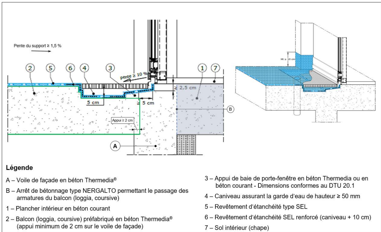
Figure n° E5-2 – Exemple de balcon, loggia ou coursive préfabriqué avec étanchéité par un S.E.L. directement circulaire - Seuil avec caniveau – 1,5 % \leq pente \leq 5 %
