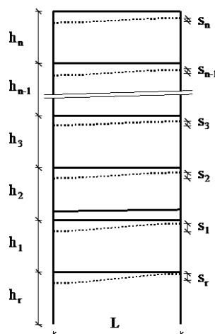
Figure 1 – Calcul des sollicitations additionnelles liées au raccourcissement relatif des murs
