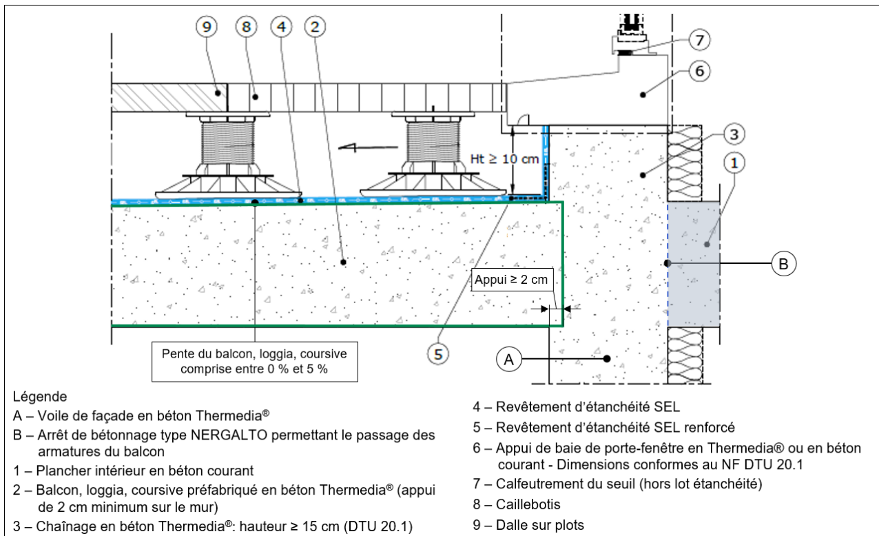
Figure n° E3-2 - Exemple de balcon, loggia ou coursive préfabriqué avec étanchéité par un S.E.L. avec protection par dalles sur plots - Seuil avec relevé de 10 cm de hauteur.
